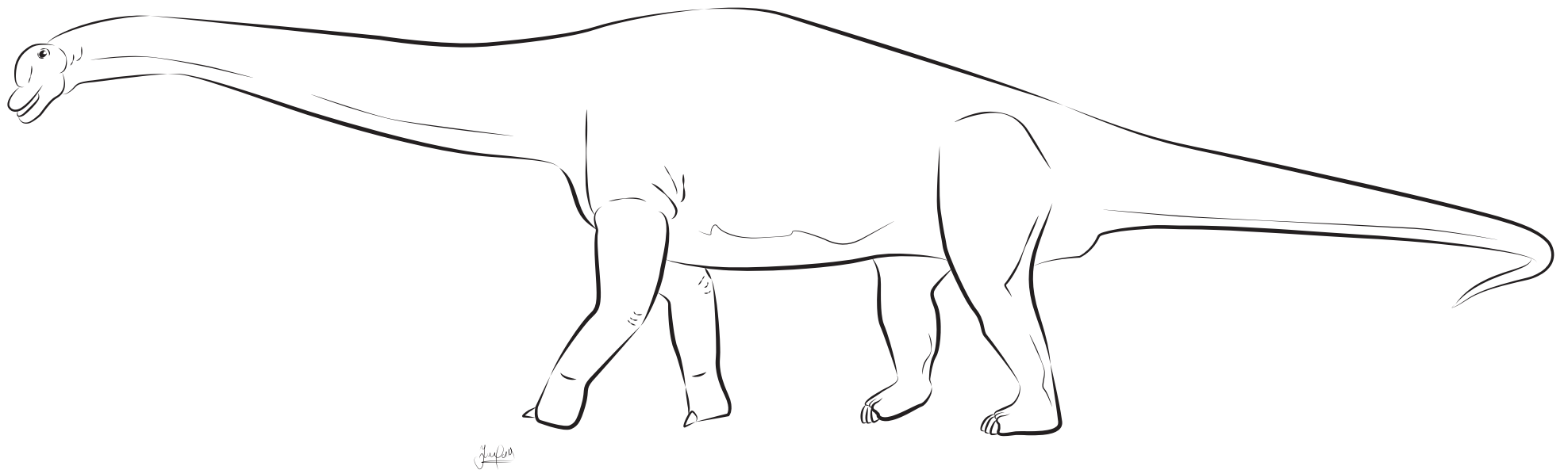
Tastavinsaurus sanzi
